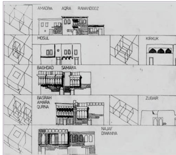
الشكل (3) تفاصيل علاقة الباحة بالبيت في انماط بيوت تقليدية في العراق. المصدر: برنامج الاسكان العام، 1982، ص 183
