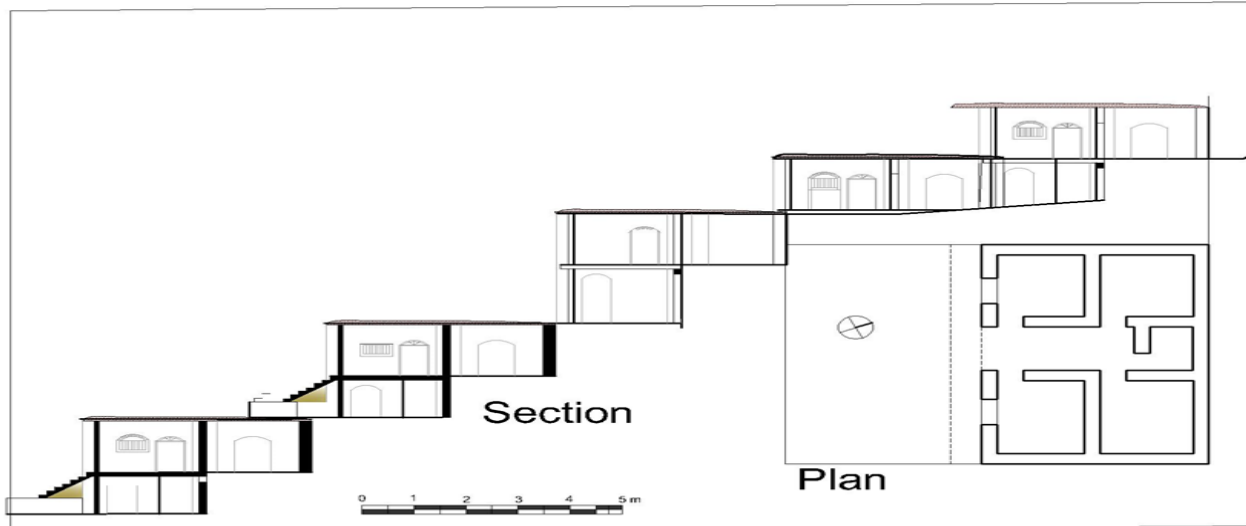
الشكل (8) تفاصيل مقطع نموذج قرية جبلية في اقليم كردستان العراق مع مخطط ل احد البيوت القروية المصدر: اعداد الباحث اعتمادا على الملاحظة الميدانية.
